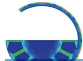
Optymalizowana struktura pola magnetycznego silnika
