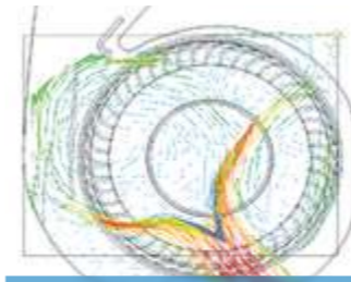
Konstrukcja równomiernego rozprowadzenia powietrza
